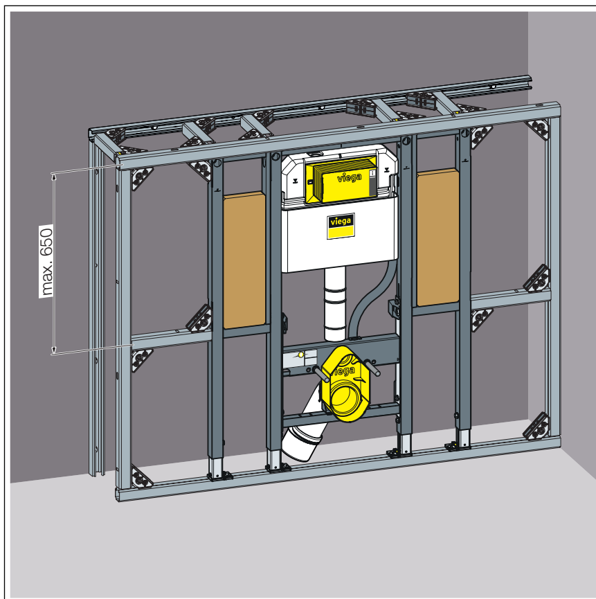
5. ábra: Akadálymentesített szerelés, 1. változat
