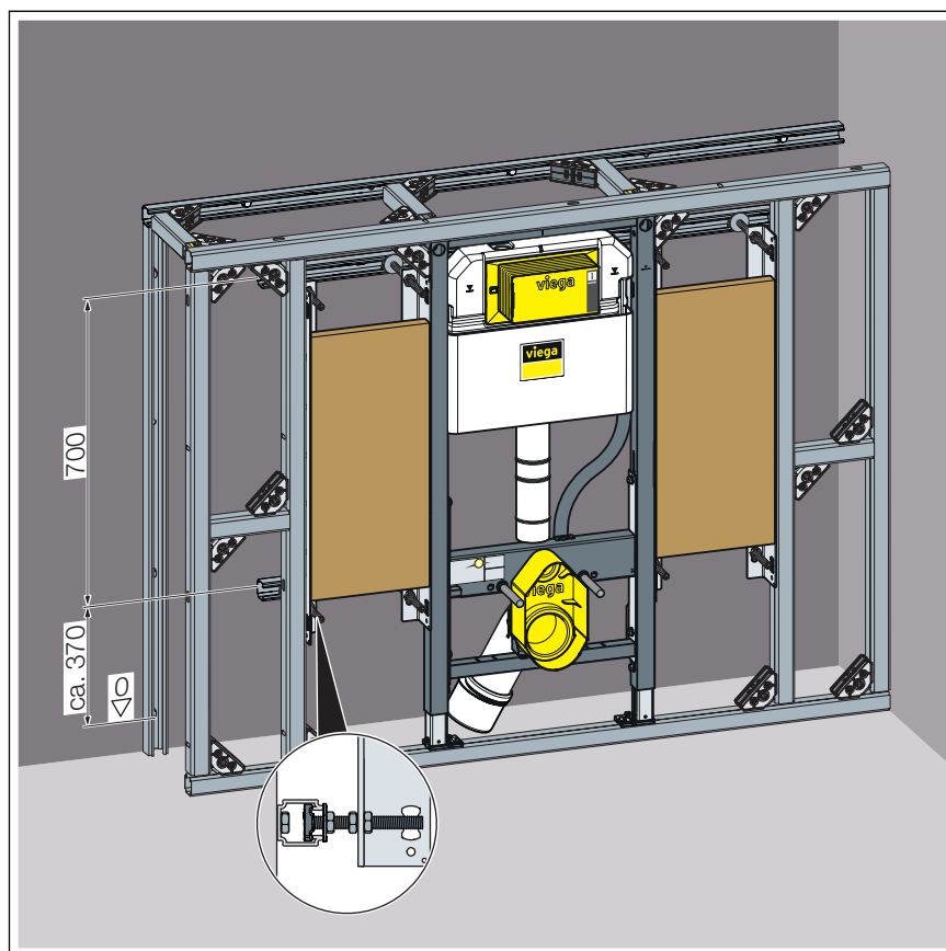
6. ábra: Akadálymentesített szerelés, 2. változat
