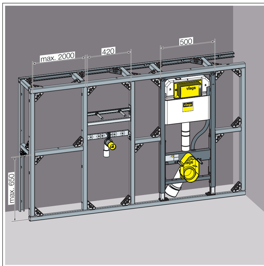
19. ábra: Függőleges sínek távolsága
