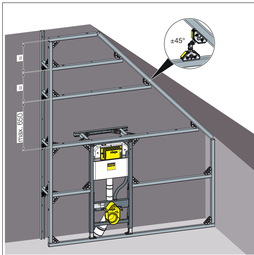
15. ábra: Beépítési méretek ferdetetűn levő előfalhoz
