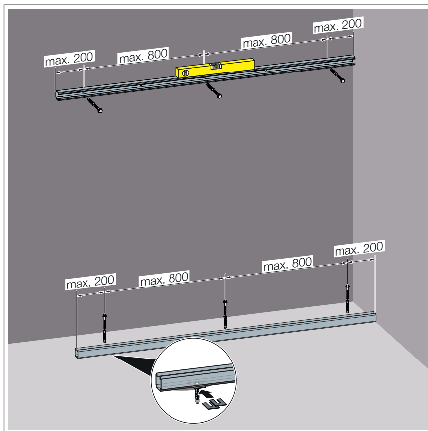
31. ábra: A sínrögzítés méretei
