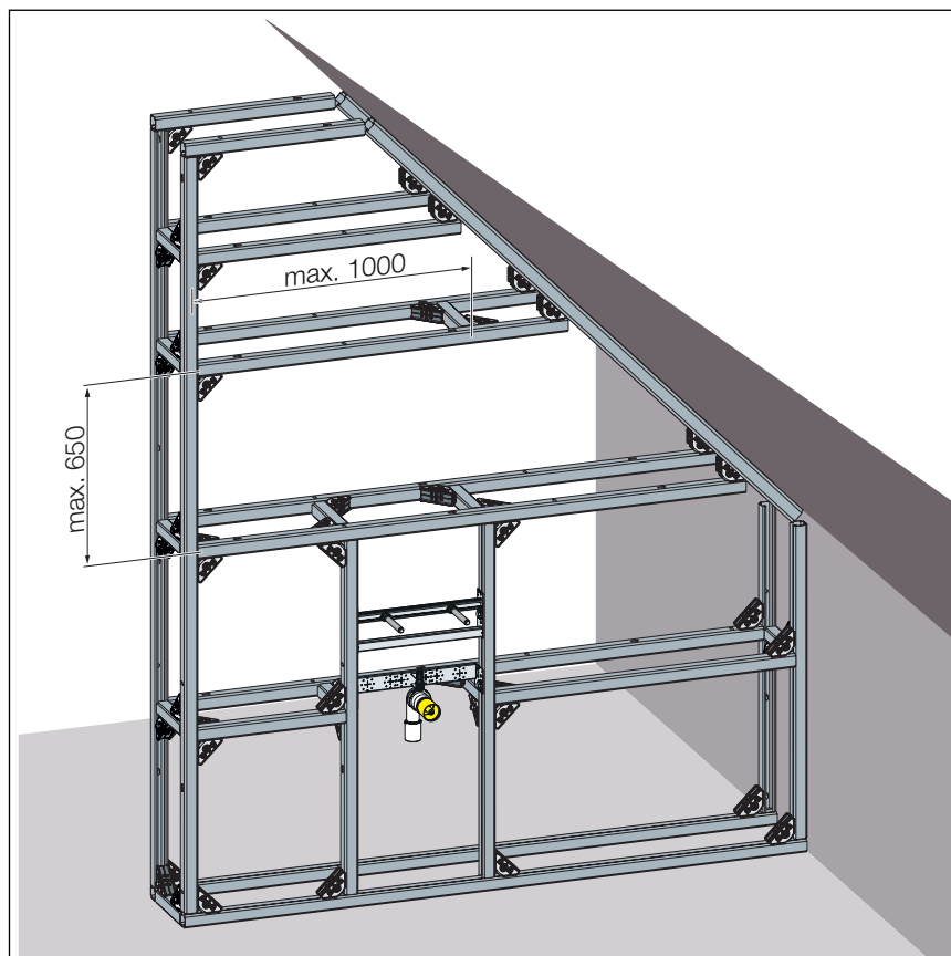
16. ábra: Beépítési méretek ferdetetőn levő válaszfalhoz
