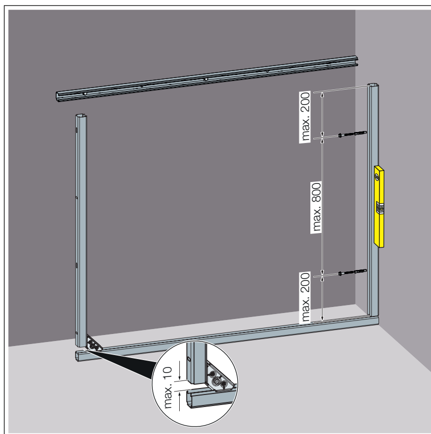
32. ábra: A sínrögzítés méretei
