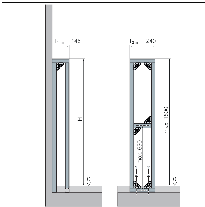
24. ábra: Félmagas előfal
