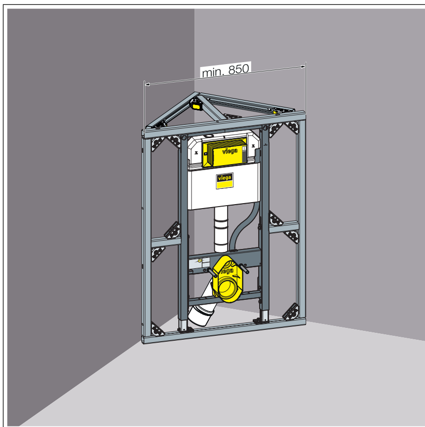
7. ábra: Sarokszerelési beépítési méretek
