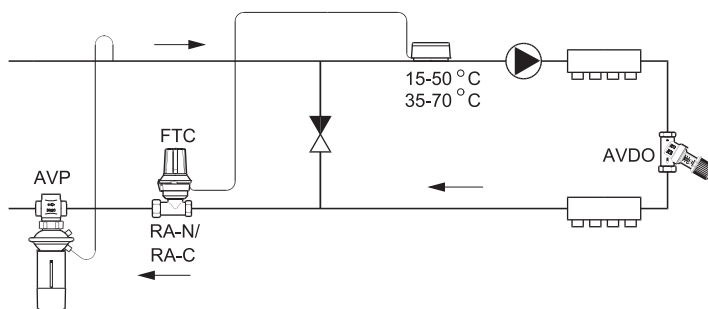
Padlófűtés direkt kapcsolással
