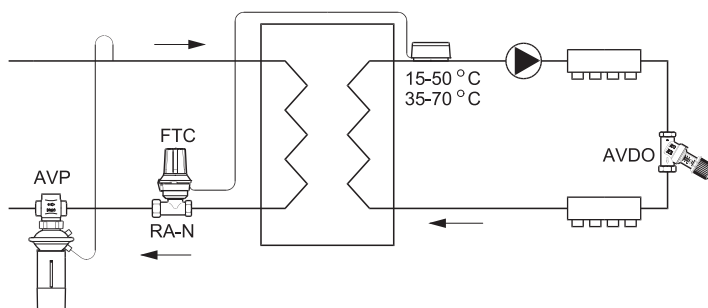
Padlófűtés hőcserélővel a radiátoros és a padlófűtési kör között
