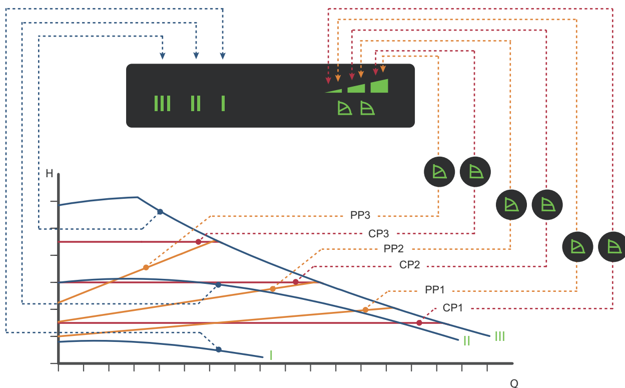
27. ábra A vezérlési funkciók és a rendszerkövetelmények kapcsolata
