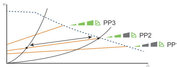
24. ábra Három arányos-nyomás jelleggörbe és beállítások
