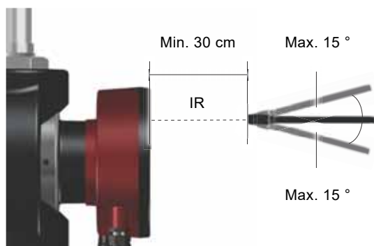
29. ábra Kapcsolat létesítése a Grundfos GO és a MAGNA1 között infravörös kommunikációval
