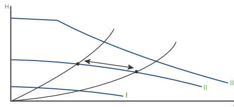
26. ábra Három állandó-görbe beállítása
