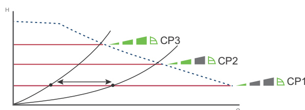
25. ábra Három állandó-nyomás jelleggörbe és beállítások
