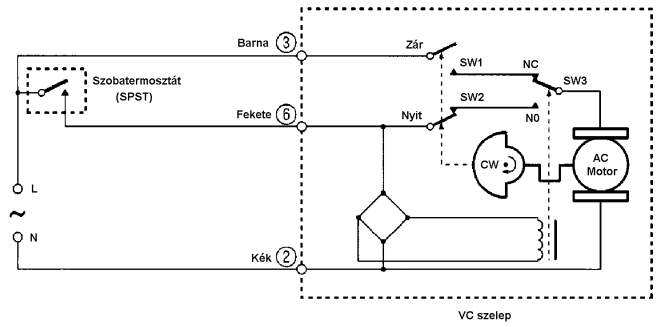
4. ábra SPST szabályzó és 2 vezetékes + fix fázis motor kapcs.
