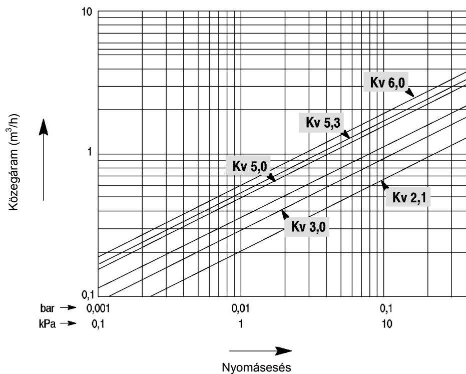
8. ábra 2-járatú szelepek kapacitás diagramja
