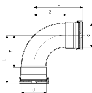
Temponox XL 90°-os ív - rozsdamentes acél modellszám 1716XL
