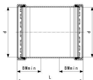
Temponox XL áttolókarmantyú - rozsdamentes acél modellszám 1715.5XL
