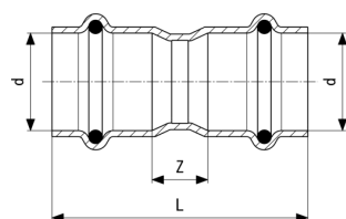
Temponox karmantyú - rozsdamentes acél modellszám 1715
