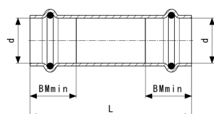
Temponox áttoló karmantyú - rozsdamentes acél modellszám 1715.5
