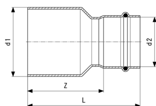
Temponox XL szűkítőidom - rozsdamentes acél modellszám 1715.1XL
