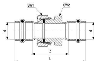
Temponox csavarzat - rozsdamentes acél modellszám 1760
